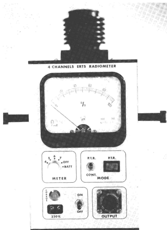
Fig. 124 - Radiometer
