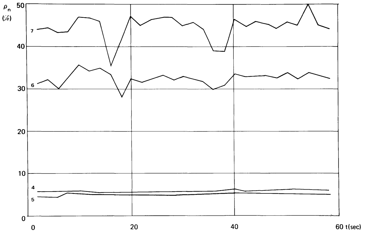
Fig. 122 - Reflectance ( Salix alba )
