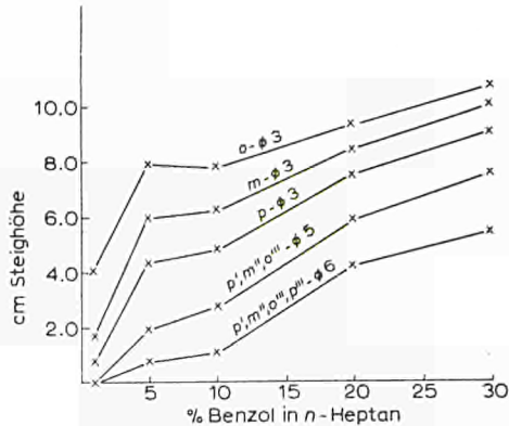
Fig. 7. Einfluss der Benzolkonzentration im Eluens (Schematische Chromatogramme). Sorbens: \text{Al}_2\text{O}_3 .
