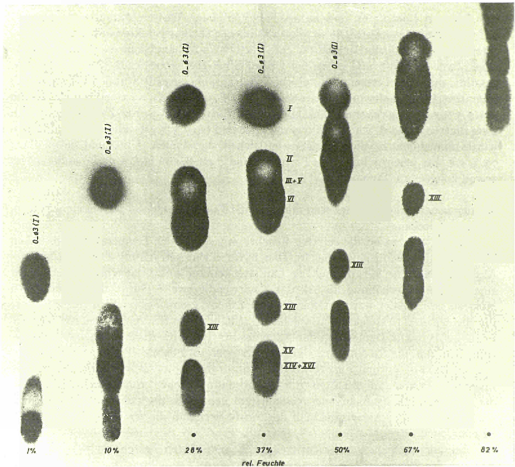
Fig. 3. Isotherme Trennung eines Polyphenyltestgemisches bei verschiedenen Klimata (Photomontage). Aufgetragene Menge/Startpunkt 0,5 \gamma insgesamt. Eluens: n -Heptan; Sorbens: \text{Al}_2\text{O}_3 , Merck; Sichtbarmachung: Besprühen mit 0,2\% iger \text{Ce}(\text{SO}_4)_2 -Lösung in konz. \text{HNO}_3 ; Photographie im U.V.-Licht 366 \text{ m}\mu . Die Platten wurden 24 Stunden vorklimatisiert und bei der jeweils gleichen Feuchte auch eluiert.
