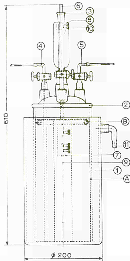
Fig. 9. Kleine Klimakammer. Handhabung siehe Praktischer Teil. 1 = Zylindrisches Entwicklungsgefäß aus Glas; 2 = Deckel mit 4 KPG-Hülsen; 3 = Tropftrichter; 4 = Gasleitungsrohr mit Hahn; 5 = Gasauslass mit Hahn; 6 = KPG-Welle; 7 = Muffe aus Teflon; 8 = Haltering aus Teflon; 9 = DSC-Platte; 10 = Schrauben aus Teflon zu 8; 11 = Überlauf für Thermostatflüssigkeit; A = Filterpapiereinlage an der Kammerinnenwand; B = Glasring mit Bohrung zur Verteilung des Eluens.
