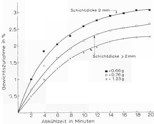
Fig. 4. Wasseraufnahme von \text{Al}_2\text{O}_3 -Schichten während des Abkühlens von 105^\circ auf 20^\circ . Schicht bei 0.76 g und 1.23 g mit dem Spatel, bei 0.66 g mit einem Streichergerät bestrichen. Raumfeuchte: 65%.
