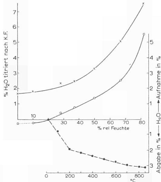
Fig. 5. Wasserhaushalt von \text{Al}_2\text{O}_3 -Schichten für DSC. (Der darin enthaltene Gips ist totgebrannt.) Oberer Teil: Isotherme Wasseraufnahme (bzw. Abnahme) in Abhängigkeit des Klimas. Linke Kurve: Wassertitration nach der Karl-Fischer-Methode (linke Ordinate). Rechte Kurve: Gewichtsmässige Wasserab- bzw. -desorption. Der Nullpunkt ist willkürlich bei 20% Gleichgewichtsfeuchte gewählt. Unterer Teil: Thermogravimetrische Messung der Wasserabspaltung bis 850^\circ (Probe bei 20% relativer Feuchte vorklimatisiert.)
