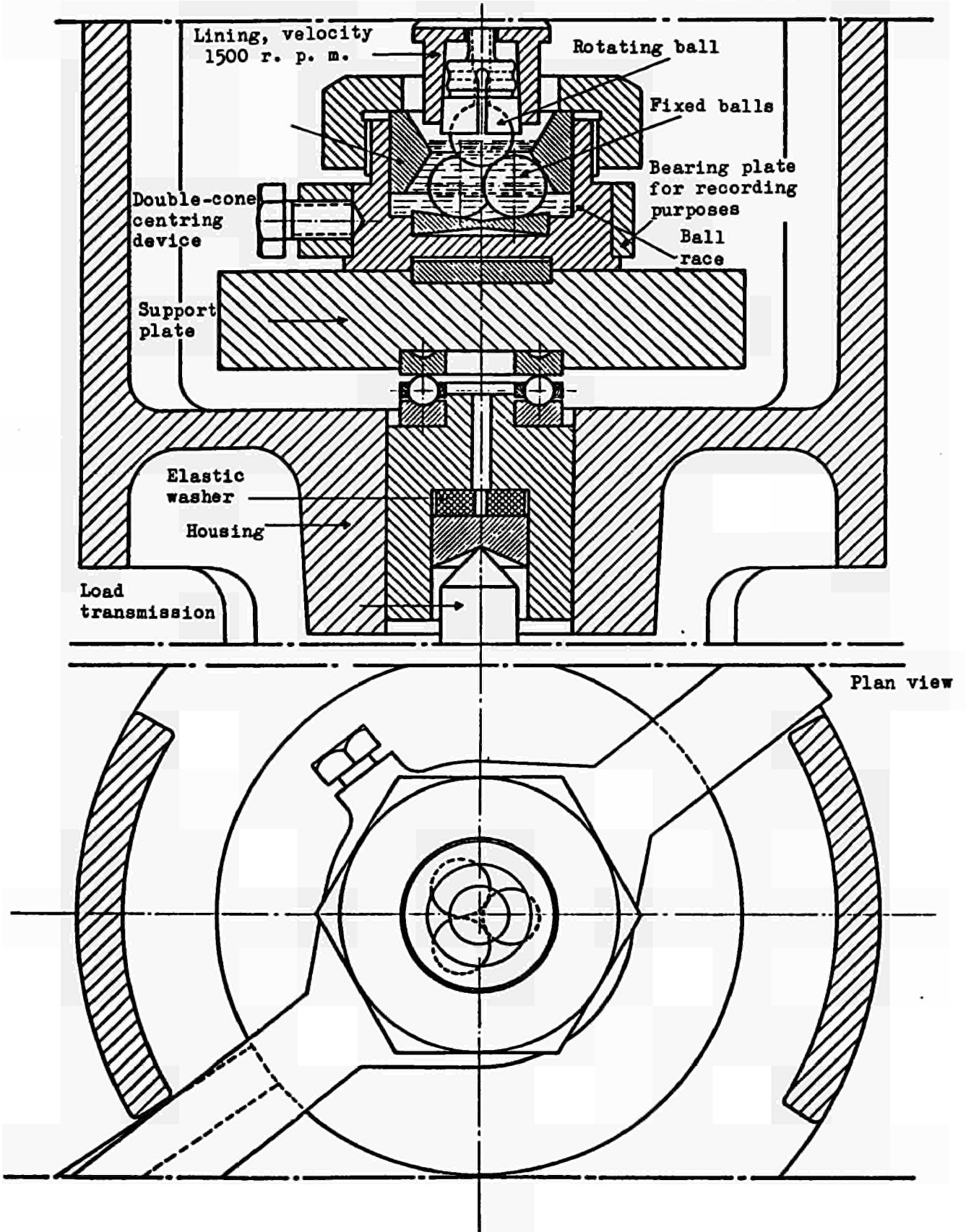
4-Ball apparatus Scale 1:1
