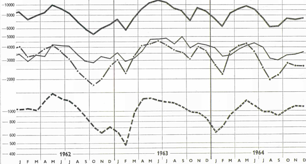
Nettoerzeugung von Primärenergie (Wasserkr. + Erdw. + Kerneng.) Production nette d'électricité primaire (Hydraul. + Géoth. + Nucléaire)
